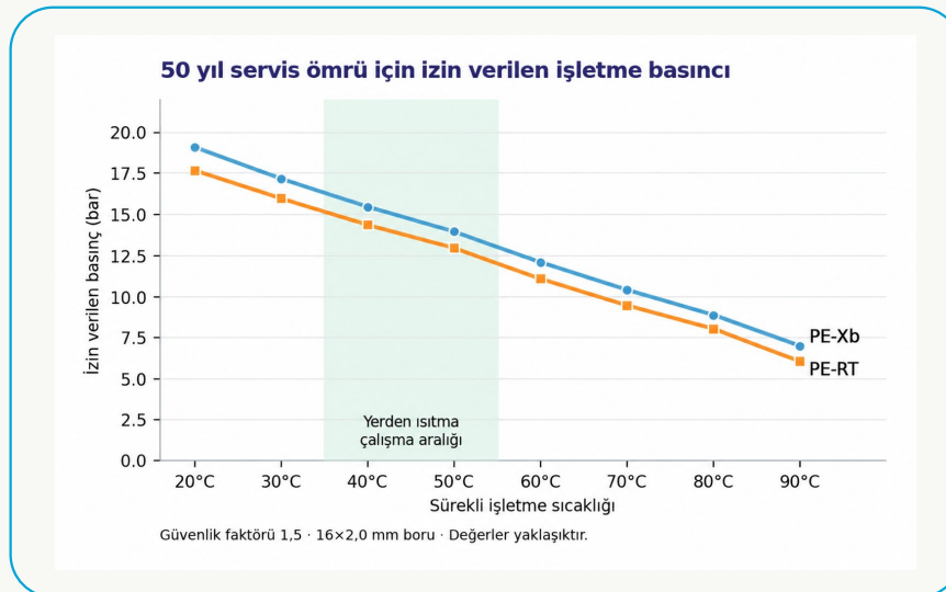
Şekil 2.1 50 yıl servis ömrü için izin verilen işletme basıncı (16×2,0 mm)
