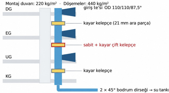
Şekil 4.3 – Fraunhofer IBP P12 test tesisindeki montaj düzeni
