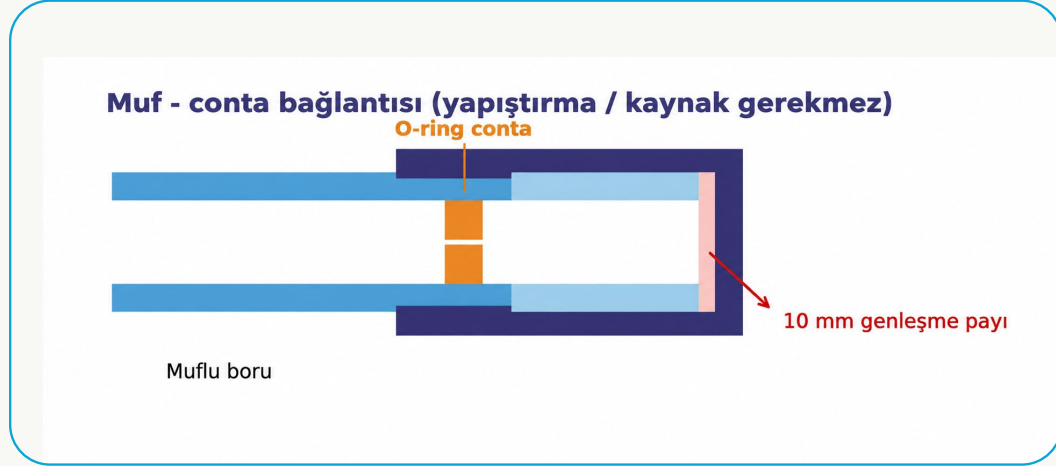
Şekil 3.1 Muf ve o-ring conta ile birleştirme
