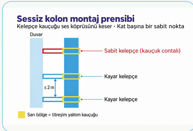
Şekil 4.4 – Sessiz kolon montaj prensibi
