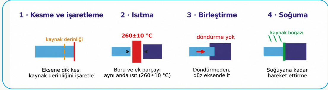
Şekil 1.5 – Polifüzyon kaynağının aşamaları
