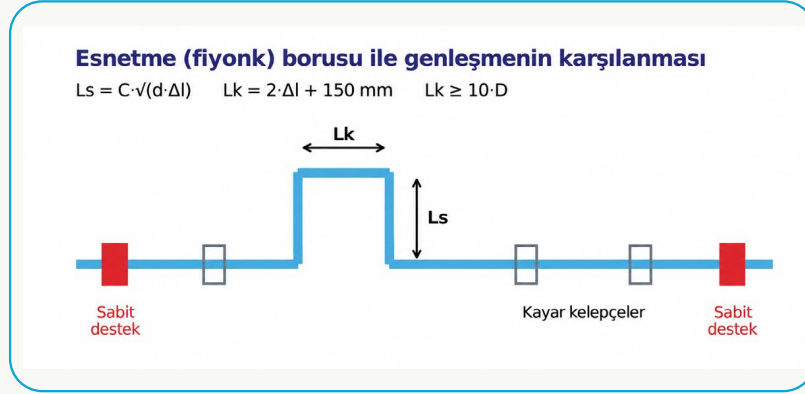
Şekil 1.4 – Esnetme (fiyonk) borusu ile genişlemenin karşılanması
