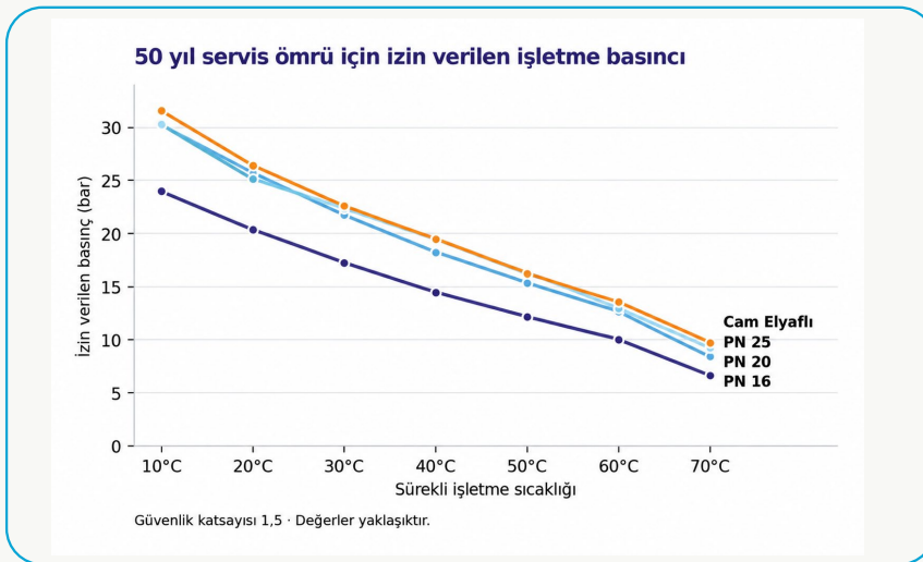
Şekil 1.2 – 50 yıl servis ömrü için izin verilen işletme basıncı
