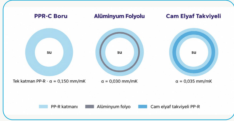
Şekil 1.1 – PPRC boru tiplerinin katman yapısı
